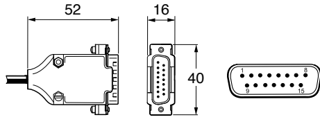
15针D型插头 (端子代码L)
