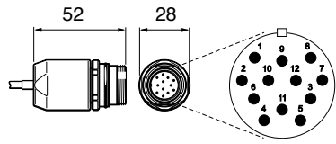
12针圆形插头 (端子代码W)
