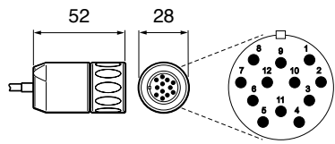
12针圆形插头 (端子代码V)
